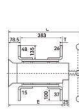
ATS 4P -3200A รุ่น HYCG1-3200 Dimension
